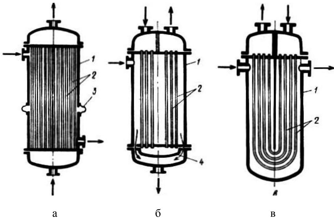
Рис.2.2.Теплообменники с компенсацией температурных напряжений корпуса 1 и теплообменных труб 2: а-с линзовыми компенсаторами 3(ТК), б-с нижней плавающей головкой 4 (ТП), в- U-образными трубками 2 (ТУ)
