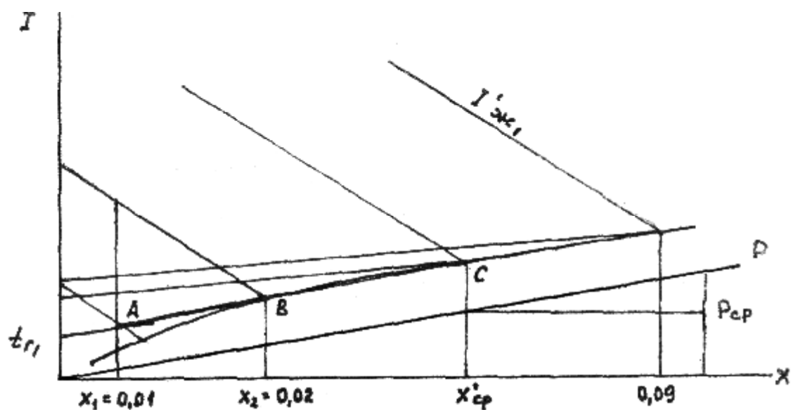
Рис.3.3. К расчету градирни локального водооборота
