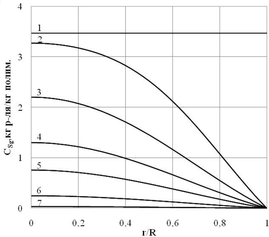
Рис. 3.11. Изменение поля концентрации растворителя внутри полимерной частицы во времени процесса при R_k=38 мм рт.ст., t_t=65 °С: 1 – \tau/\tau_{пр}=0 ; 2 – \tau/\tau_{пр}=0,1 ; 3 – \tau/\tau_{пр}=0,2 ; 4 – \tau/\tau_{пр}=0,3 ; 5 – \tau/\tau_{пр}=0,4 ; 6 – \tau/\tau_{пр}=0,6 ; 7 – \tau/\tau_{пр}=1
