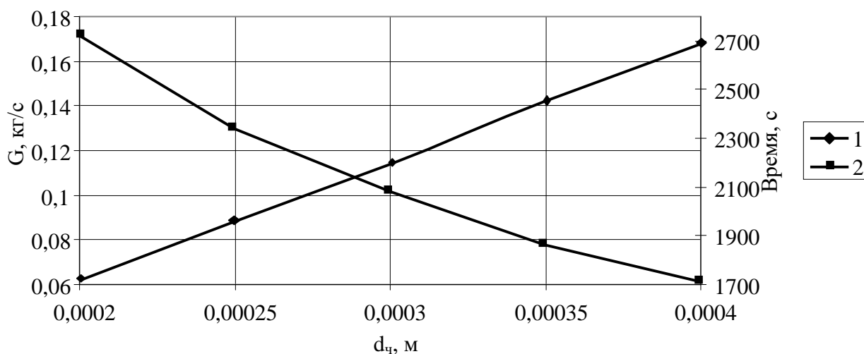
Рис. 5.10. Зависимости расхода воздуха (1) и времени процесса сушки (2) от размера частиц порошка: d_{ап} = 0,8 \text{ м} ; K_w = 0,7
