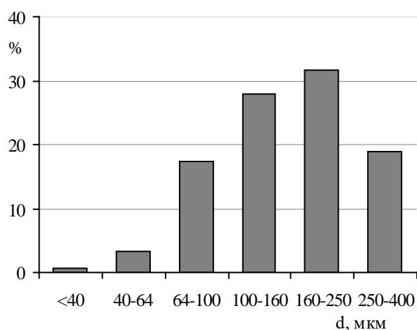
Рис. 4.9. Дисперсный состав полимерного порошка, полученного из опыта с параметрами: t_{ст(б)}=55\text{ }^{\circ}\text{C} ; C_p=40\text{ }% ; n=25\text{ об/мин}
