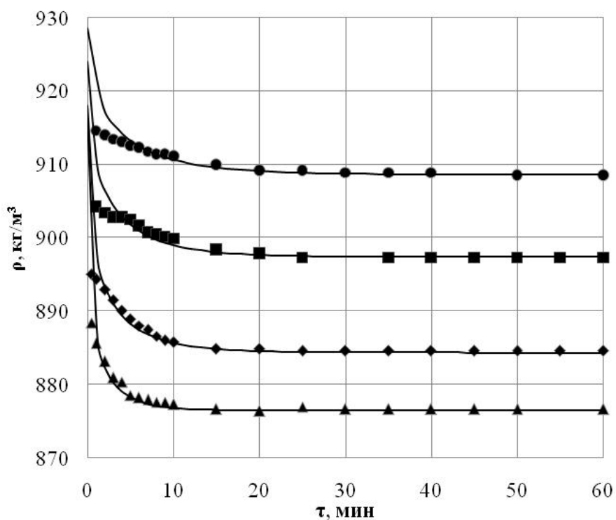
Рис. 2.8. Зависимость плотности образца в течение набухания при различных температурах: ▲ – 50°C; ◆ – 45 °C; ■ – 35 °C; ● – 25 °C
