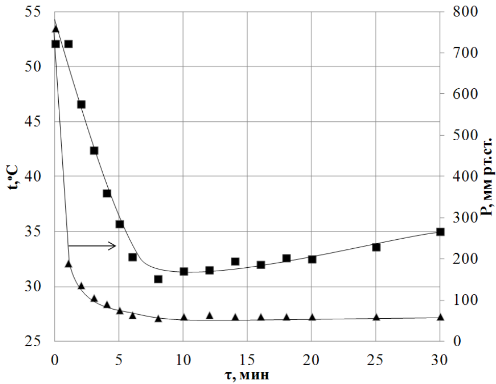
Рис. 3.3. Зависимость температуры жидкой фазы и давления в аппарате от времени процесса при наличии полимерной фазы: P_k=61 мм рт.ст., t_r=60^\circ\text{C}
