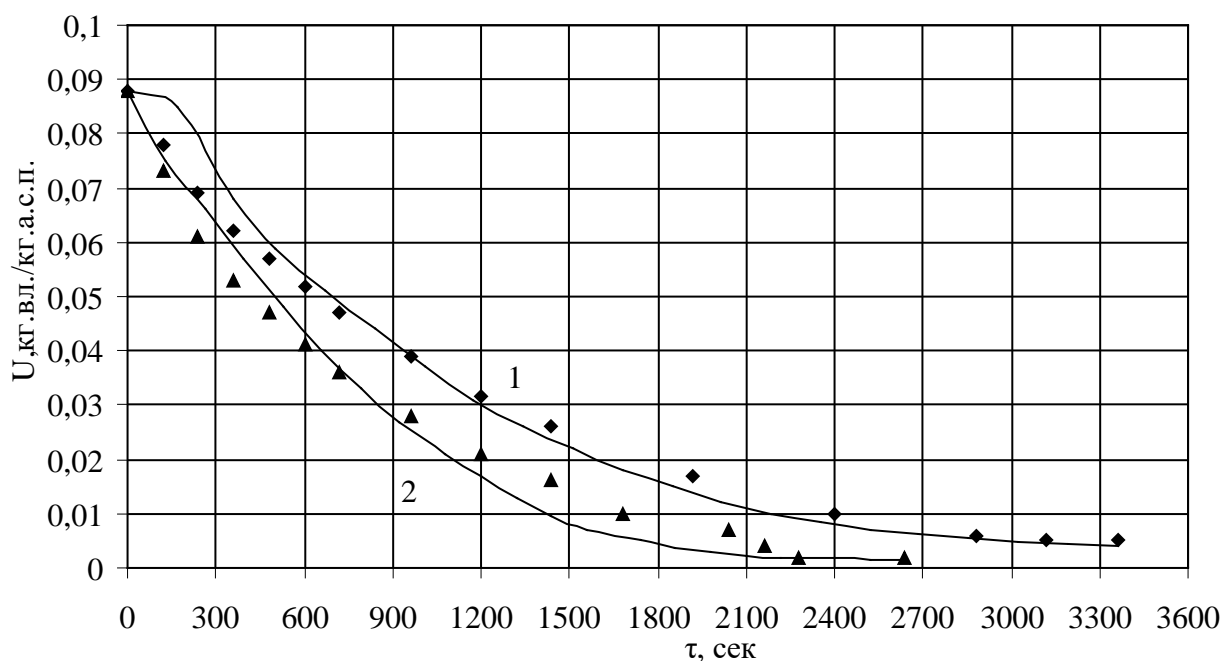
Рис. 4.56. Зависимости изменения влагосодержания полимерного порошка от времени процесса: 1 – t_r = 60 \text{ °C} ; 2 – t_r = 90 \text{ °C}
