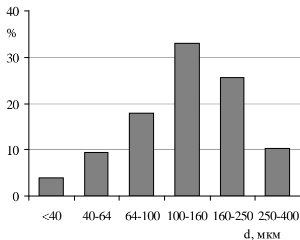
Рис. 4.9. Дисперсный состав полимерного порошка, полученного из опыта с параметрами: t_{ст(б)}=55\text{ }^{\circ}\text{C} ; C_p=40\text{ }% ; n=25\text{ об/мин}
