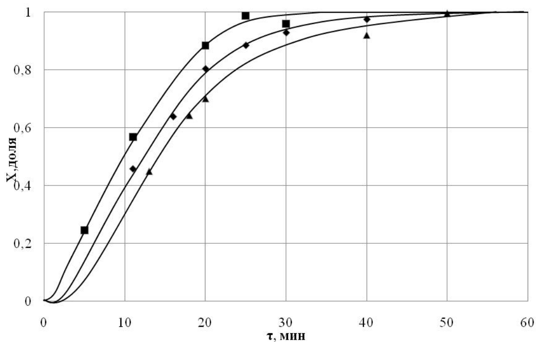
Рис. 2.14. Изменение массовой доли растворившегося полимера во времени: C_{\text{ПЭНП}} = 25\% ; n = 180 \text{ мин}^{-1} ; ▲ – t_{\text{T}} = 80 \text{ }^{\circ}\text{C} ; ◆ – t_{\text{T}} = 88 \text{ }^{\circ}\text{C} ; ■ – t_{\text{T}} = 110 \text{ }^{\circ}\text{C}
