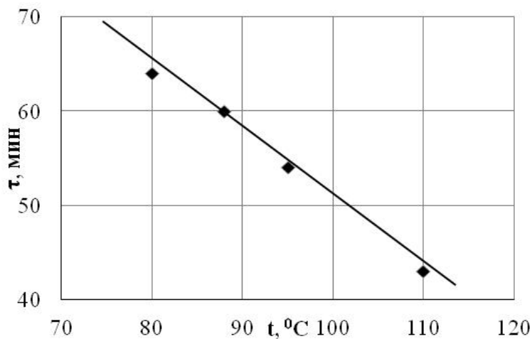
Рис. 2.17. Зависимость времени растворения от температуры теплоносителя:
