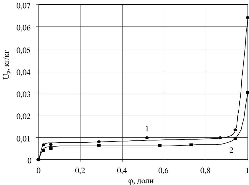
Рис. 5.11. Изотермы сорбции и десорбции для порошка полиэтилена t = 20\text{ }^\circ\text{C} : 1 - кривая десорбции; 2 - кривая сорбции
