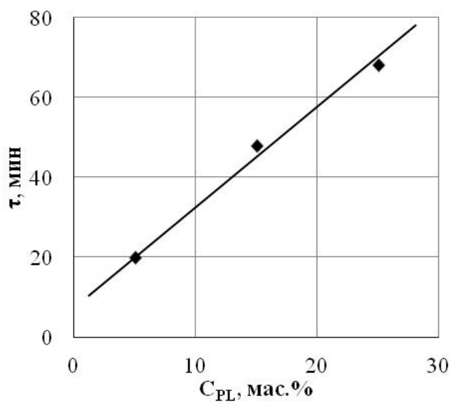
Рис. 2.16. Зависимость времени растворения от концентрации приготавливаемого раствора: t_{\text{T}} = 95\text{ }^{\circ}\text{C} ; n = 130\text{ мин}^{-1}
