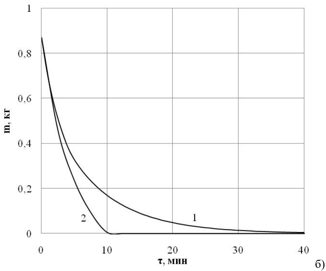
Рис. 3.7. Изменение температуры (а) и массы (б) растворителя во времени процесса для системы полимер – растворитель – вода (1) и растворитель – вода (2): R_k=38 \text{ мм рт.ст.} , t_t = 70 \text{ }^\circ\text{C}
