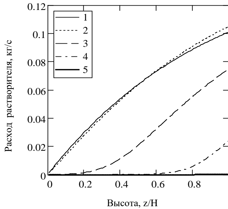
Рис. 4.37. Зависимости изменения расхода растворителя по высоте аппарата с различной продолжительностью процесса.
