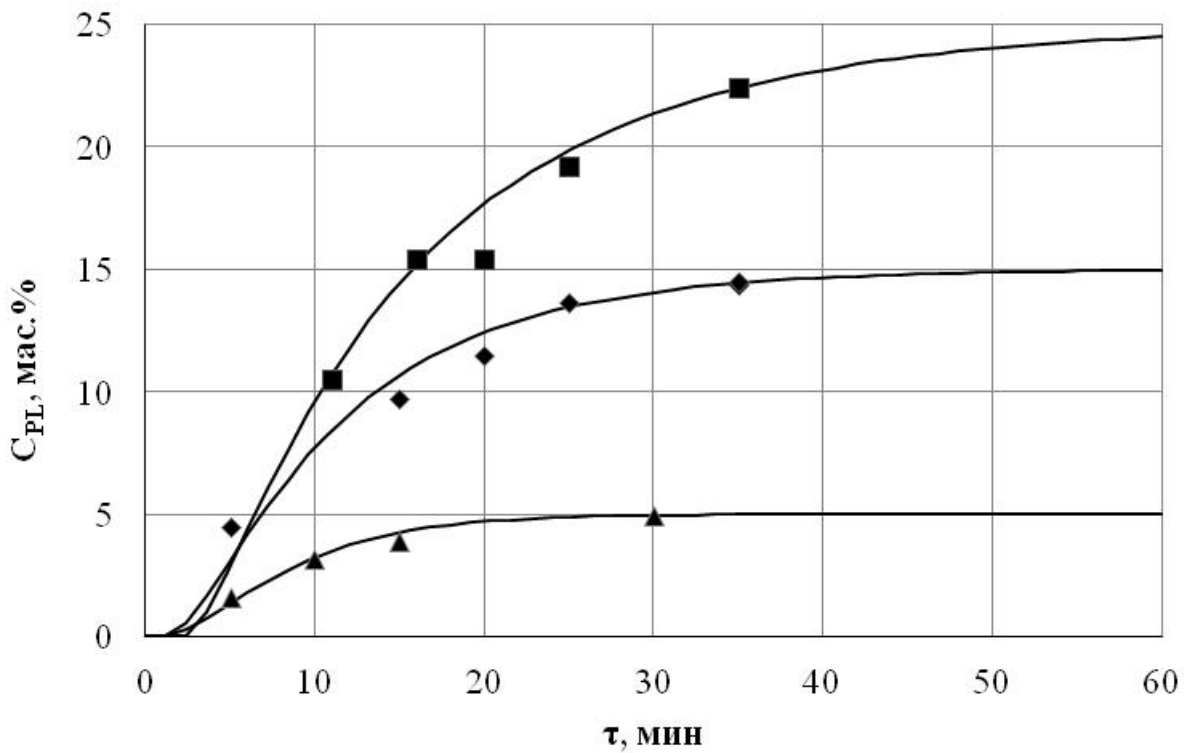
Рис. 2.20. Изменение концентрации полимера в растворе во времени: t_r=95\text{ }^{\circ}\text{C} ; n=130\text{ мин}^{-1} ; ▲ – C_{\text{ПЭНП}}=5\% ; ◆ – C_{\text{ПЭНП}}=15\% ; ■ – C_{\text{ПЭНП}}=25\%
