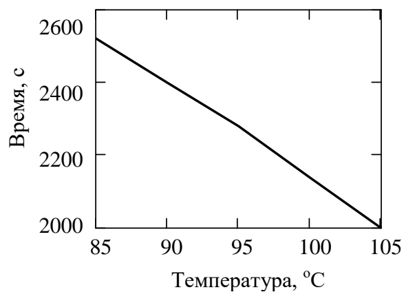
Рис. 4.57. Зависимость длительности процесса сушки от температуры сушильного агента
