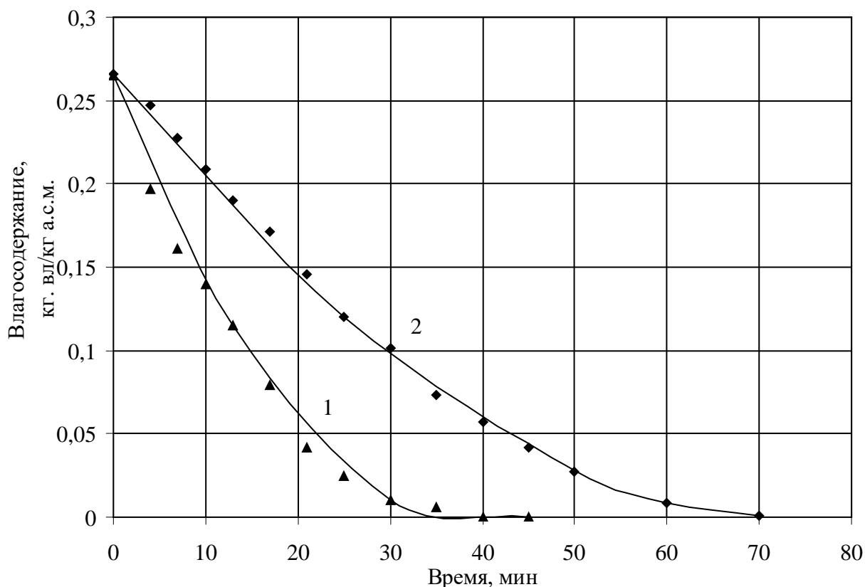
Рис. 4.46. Кривые сушки порошка полиэтилена при P = 0,6 атм: 1 - t = 80 °C; 2 - t = 60 °C
