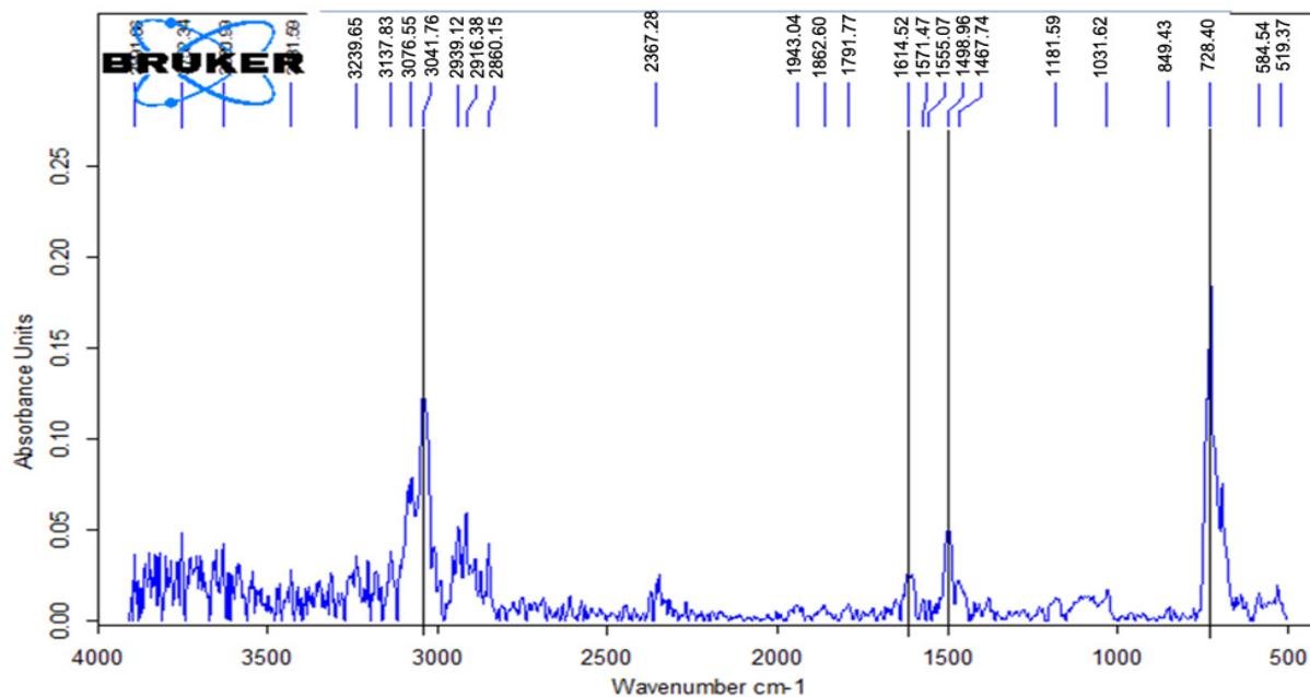
Рис. 4.26. ИК-спектр полимерного порошка перед процессом удаления растворителя; t = 50\text{ }^{\circ}\text{C}
