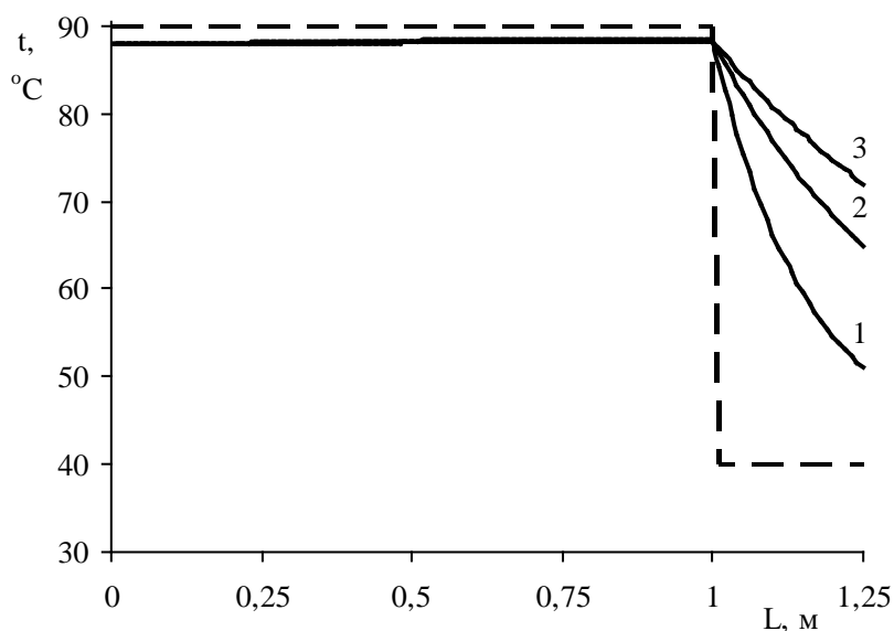
Рис. 5.5. Распределение температуры раствора полимера по длине аппарата при различных оборотах рабочего органа: 1 – n=20 мин -1 ; 2 – n=45 мин -1 ; 3 – n=70 мин -1
