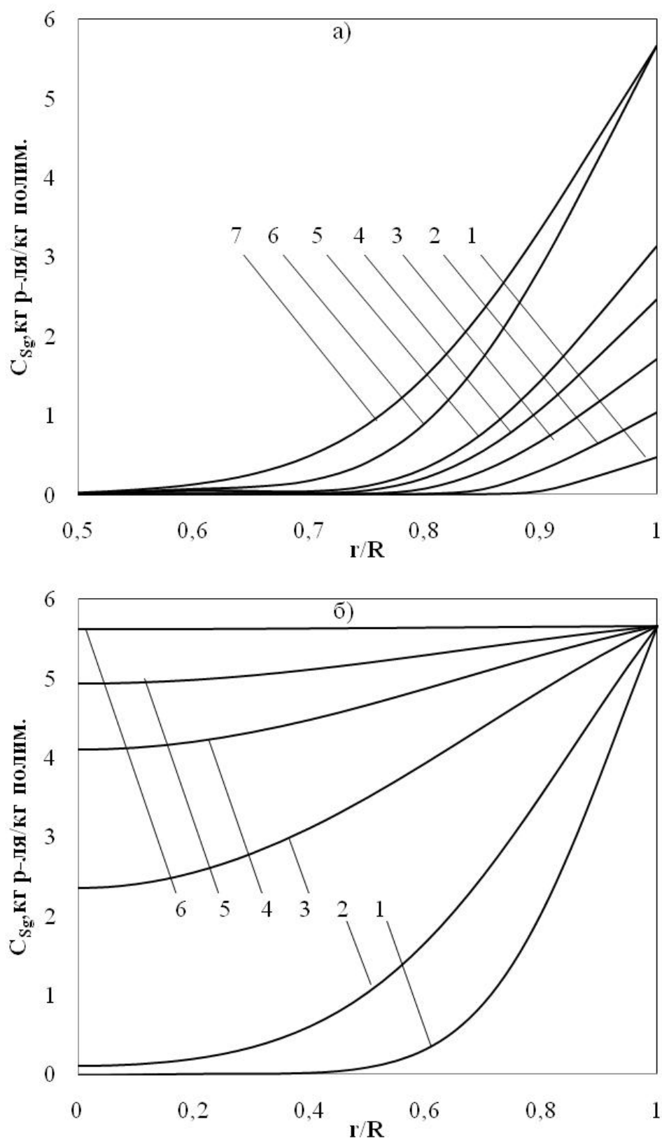
Рис. 2.24. Изменение поля концентрации растворителя в грануле во времени процесса при C_{ПЭНП}=15\% ; t_r=95 °С; n=130 мин -1 ; d=4 мм: а) 1 – \tau=10 с; 2 – \tau=70 с; 3 – \tau=90 с; 4 – \tau=100 с; 5 – \tau=105 с; 6 – \tau=120 с; 7 – \tau=150 с; б) 1 – \tau=3 мин; 2 – \tau=5 мин; 3 – \tau=10 мин; 4 – \tau=15 мин; 5 – \tau=20 мин; 6 – \tau=40 мин
