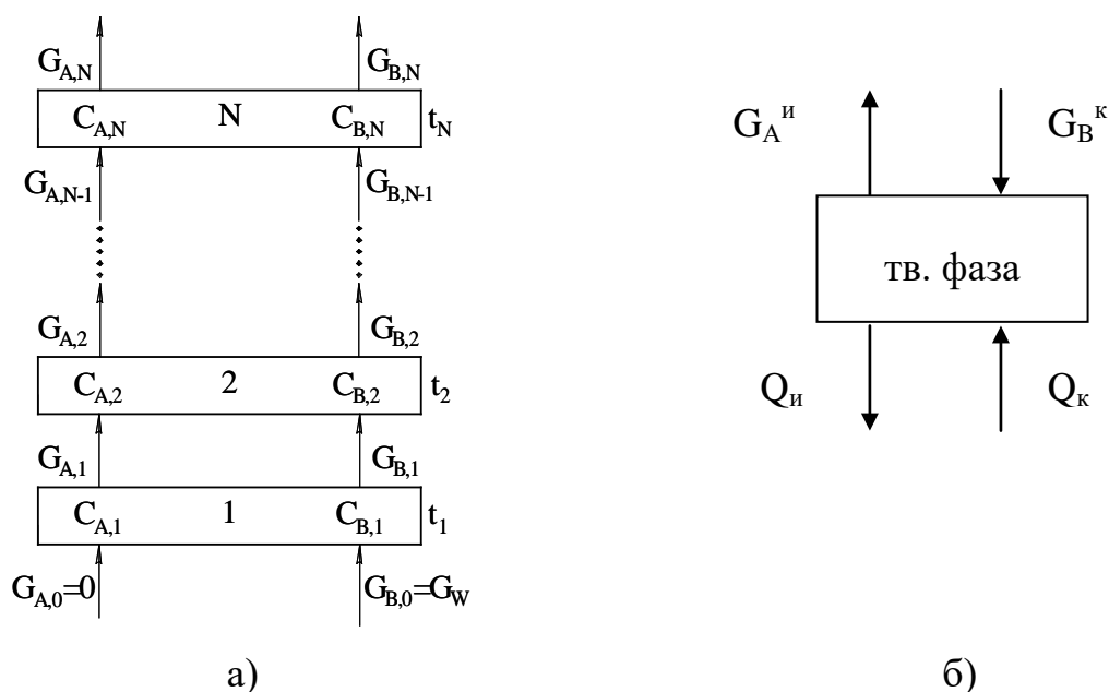
Рис. 4.28. Расчётные схемы к составлению системы уравнений материальных и тепловых балансов: G_A^И - расход испарившегося растворителя; G_B^К - расход сконденсировавшихся водяных паров; Q_И - теплота испарения; Q_К - теплота конденсации
