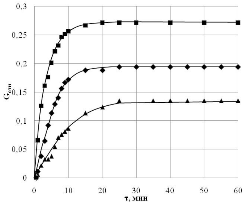
Рис. 2.6. Относительное изменение веса образца при различных температурах процесса: ▲ – 35 °С; ◆ – 45 °С; ■ – 55 °С
