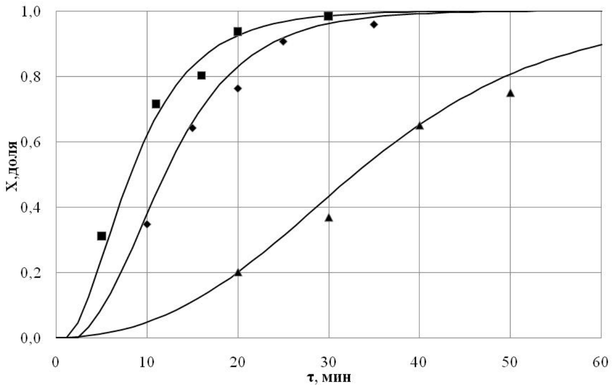
Рис. 2.21. Изменение массовой доли растворившегося полимера во времени: C_{\text{ПЭНП}}=15\% ; t_r=95\text{ }^{\circ}\text{C} ; ▲ – n=30\text{ мин}^{-1} ; ◆ – n=130\text{ мин}^{-1} ; ■ – n=180\text{ мин}^{-1}
