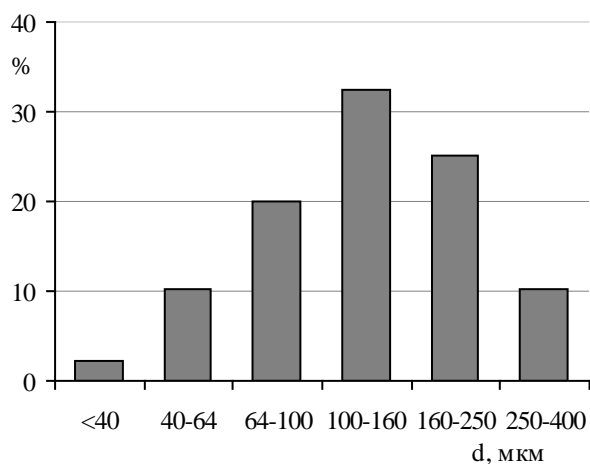
Рис. 4.11. Дисперсный состав полимерного порошка, полученного из опыта с параметрами: t_{ст(б)}=55\text{ }^{\circ}\text{C} ; C_p=35\text{ }% ; n=25\text{ об/мин}
