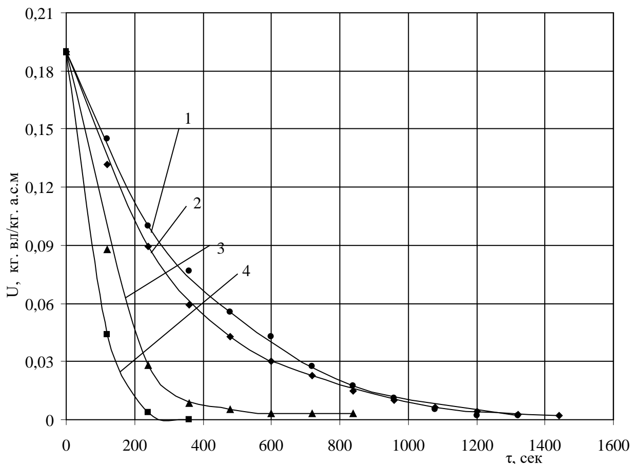
Рис. 4.48. Кривые сушки полимерного порошка. H_{сл} = 0,01 м; t_r = 65 °С:
