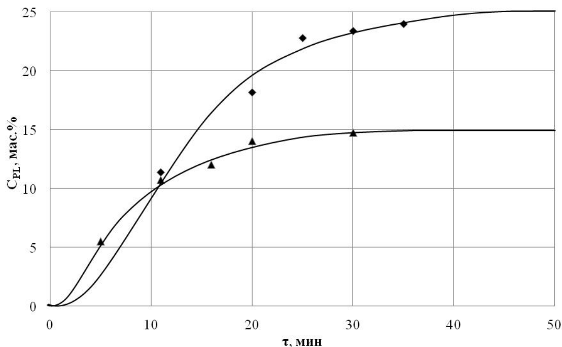
Рис. 2.13. Изменение концентрации полимера в растворе во времени: t_T=95\text{ }^{\circ}\text{C} ; n=180\text{ мин}^{-1} ; \blacktriangle – C_{ПЭНП}=15\% ; \blacklozenge – C_{ПЭНП}=25\%
