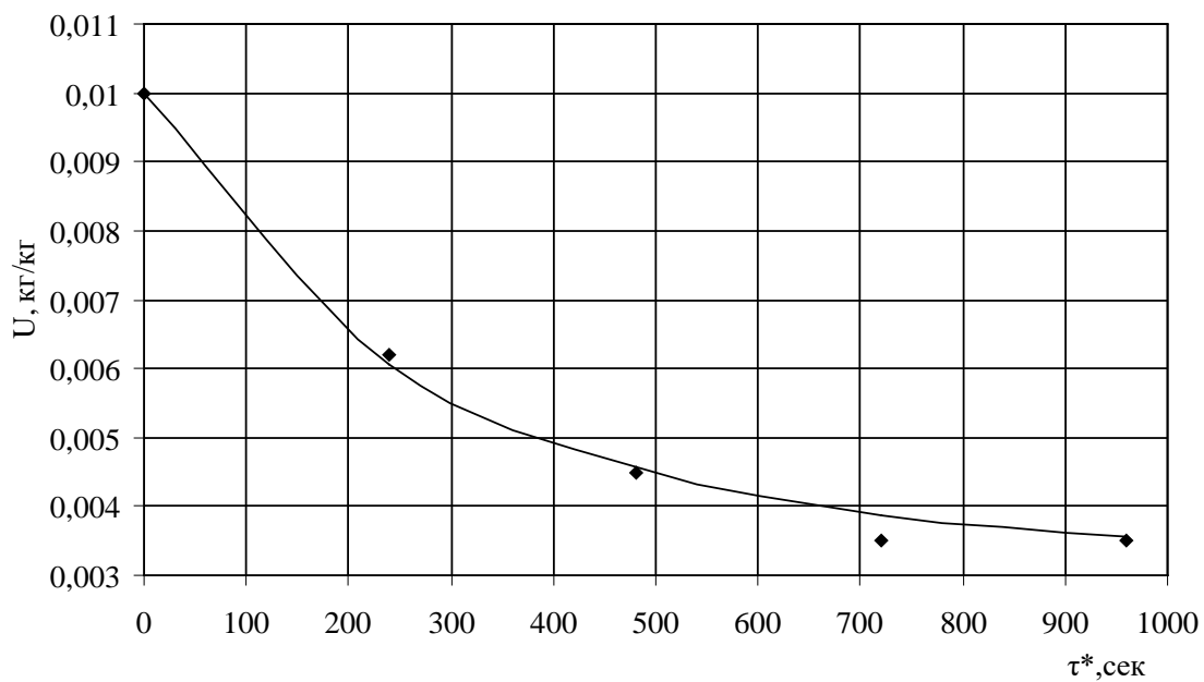
Рис. 4.53. Кривая сушки второго периода для порошка полиэтилена. Температура эксперимента t = 70\text{ °C}
