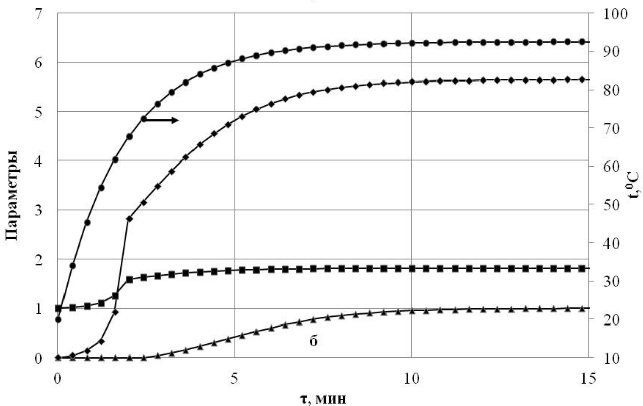
Рис. 2.23. Изменение ● – температуры системы t, ^\circ\text{C} ; ◆ – среднеобъемной концентрации растворителя в грануле C_{Sg}, \text{кг р-ля/кг полим.} ; ■ – радиуса гранулы R \cdot 10^3, \text{м} ; ▲ – доли полимера, перешедшего в раствор, масс. во времени процесса при C_{\text{ПЭНП}}=15\% , t_r=95 ^\circ\text{C} , n=130 \text{ мин}^{-1} : а) эквивалентный диаметр гранул ПЭНП d=4\text{мм} , б) d=2\text{мм} .
