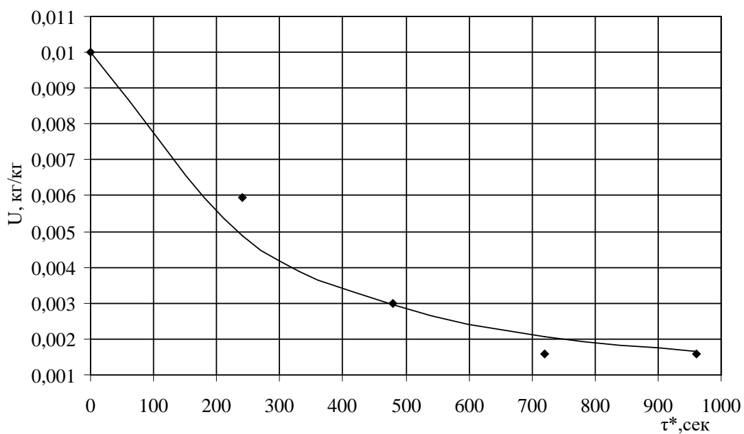
Рис. 4.54. Кривая сушки второго периода для порошка полиэтилена. Температура эксперимента t = 90\text{ °C}
