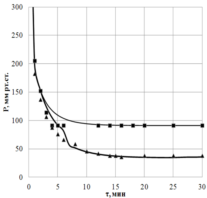
Рис. 3.8. Зависимость температуры жидкой фазы (а) и давления в аппарате (б) от времени процесса для системы полимер-растворитель-вода. Температура теплоносителя t_t=70^\circ\text{C} , давление в конденсаторе P_k : ▲ – 38 мм рт.ст; ■ – 91 мм рт.ст.
