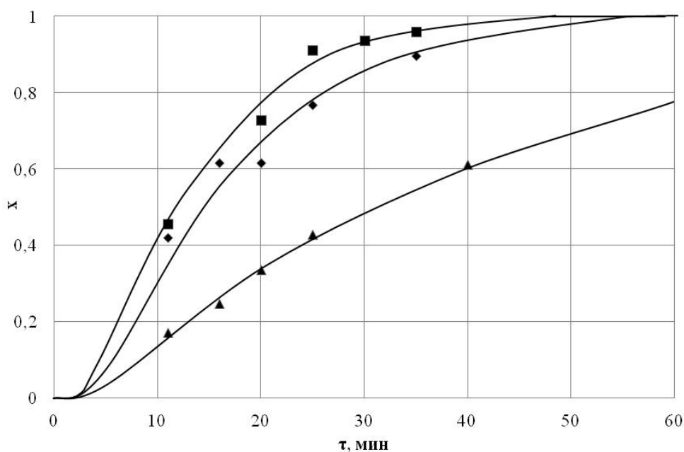
Рис. 2.15. Изменение массовой доли x растворившегося полимера во времени: C_{\text{ПЭНП}} = 25\% ; t_{\text{T}} = 95\text{ }^{\circ}\text{C} ; \blacktriangle – n = 30\text{ мин}^{-1} ; \blacklozenge – n = 130\text{ мин}^{-1} ; \blacksquare – n = 180\text{ мин}^{-1}
