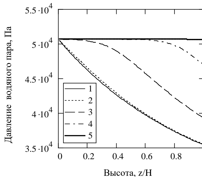
Рис. 4.34. Зависимости изменения давления водяного пара по высоте аппарата с различной продолжительностью процесса. Время, с: 1 - 160; 2 - 320; 3 - 480; 4 - 640; 5 - 800
