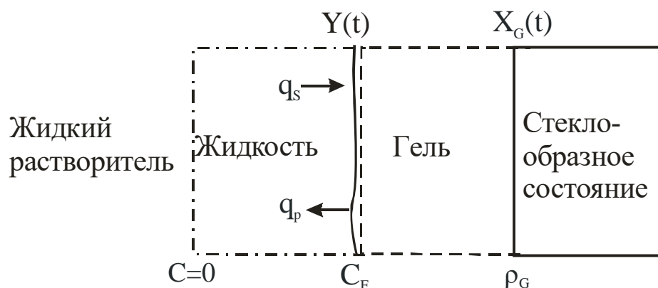
Рис.2.3. Схематическое изображение образующихся фаз в растворяющемся полимере
