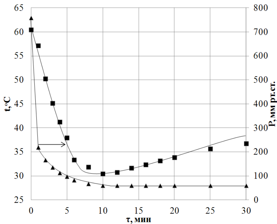
Рис. 3.4. Зависимость температуры жидкой фазы и давления в аппарате от времени процесса при наличии полимерной фазы: P_k=61 мм рт.ст., t_r=70^\circ\text{C}
