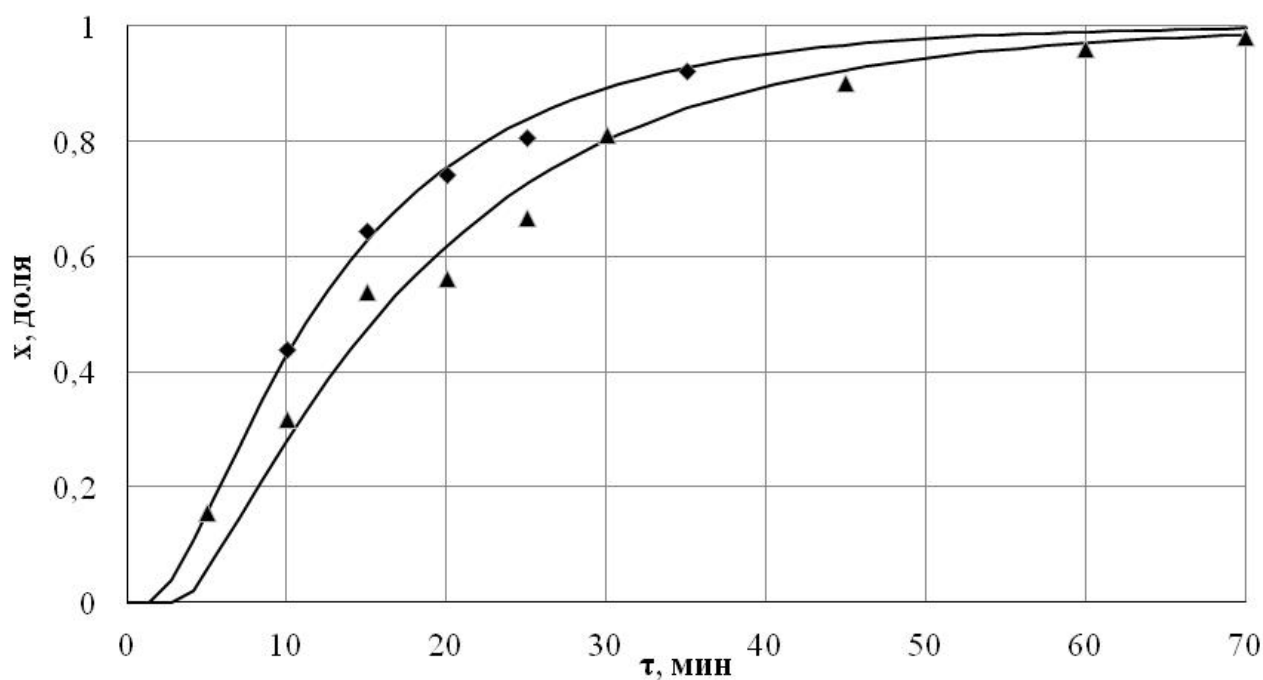
Рис. 2.22. Изменение массовой доли растворившегося полимера во времени:
