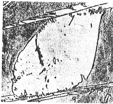
Рис. 4.9. Редкий случай расположения мартенситной пластины в плоскости шлифа. \times 750 (А.П. Гуляев, Е.В. Петунина)
