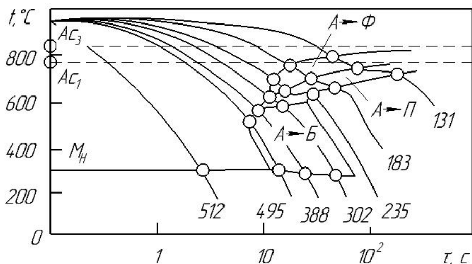
Рис. 4.16. Термокинетическая диаграмма для стали 35ГС, содержащей 0,34% С, 1% Мn, 0,76% Si (К.Ф. Стародубов, Ю.З.Борковский, В.В.Парусов)
