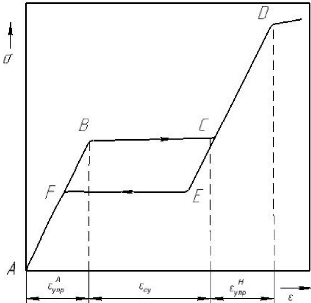
Рис. 4.13. Схема, иллюстрирующая проявление сверхупругости ( \epsilon_{\text{упр}}^A и \epsilon_{\text{упр}}^M – упругая деформация аустенита и мартенсита соответственно; \epsilon_{\text{су}} – сверхупругая деформация)
