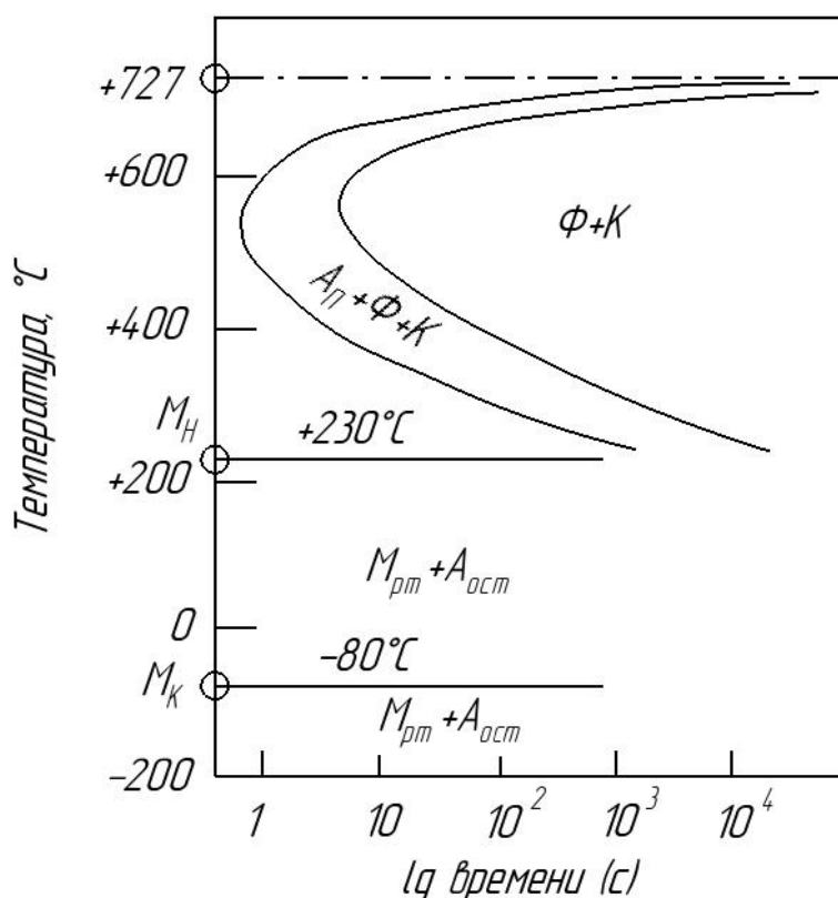
Рис. 4.2. С-диаграмма с мартенситными точками для стали с 0,8% C:
