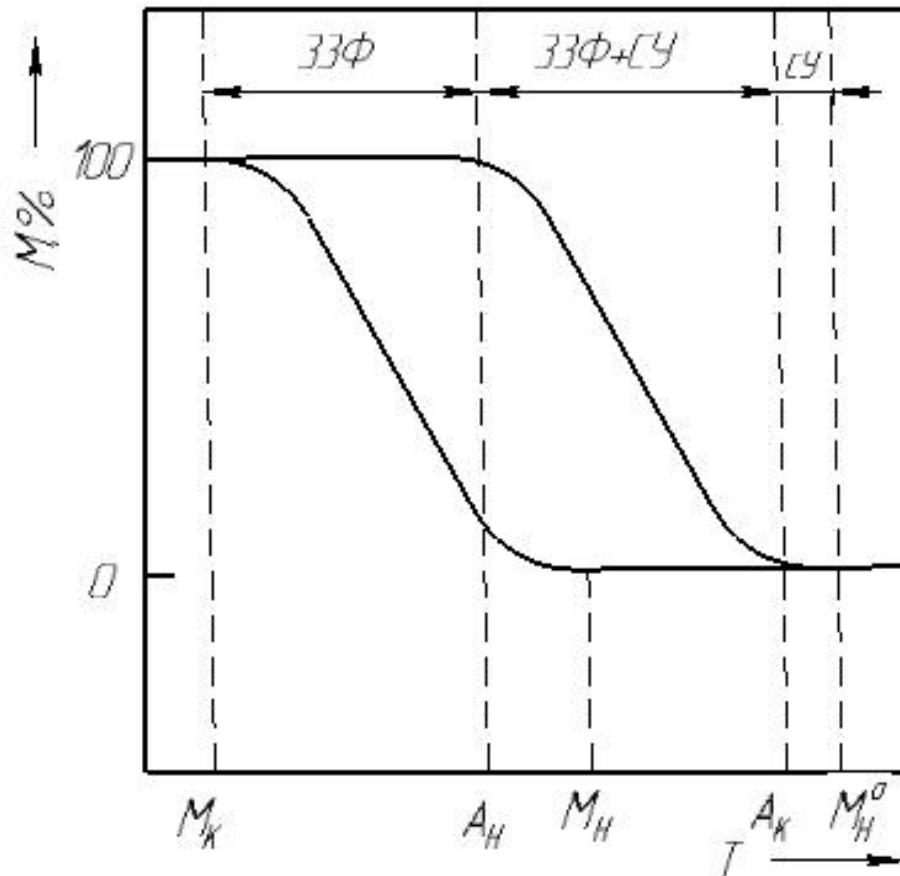
Рис. 4.12. Изменение количества термоупругого мартенсита при охлаждении и нагреве
