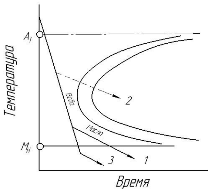
Рис. 4.20. Закалка через воду в масло (закалка в двух средах): 1 – нормальный режим; 2 – недоудержка в воде; 3 – передержка в воде
