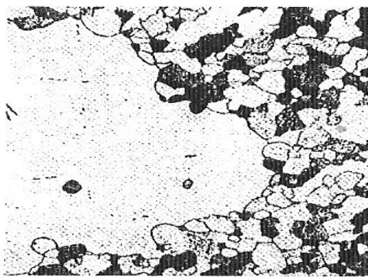
Рис. 2.7. Граница между мелкими зернами и крупным зерном, образовавшимся в цинке в результате вторичной рекристаллизации во время отжига при 200°C. х60 (Бурке)
