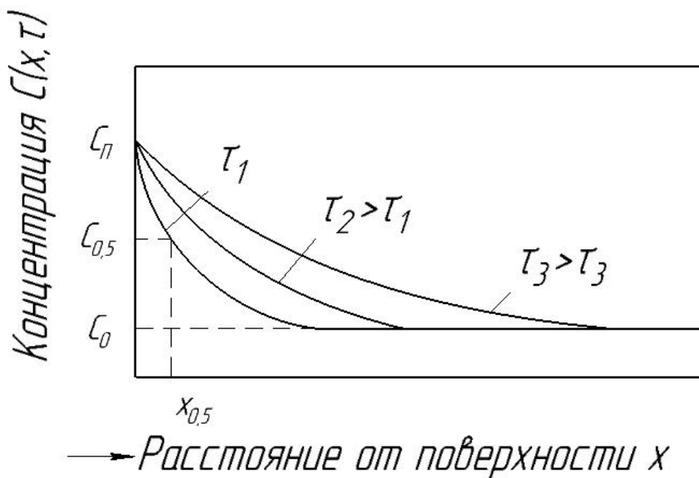
Рис. 7.1. Распределение концентрации в однофазной зоне диффузионного обогащения в разные моменты времени при постоянной концентрации на поверхности C_{\pi}
