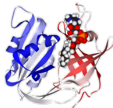
Цитохром b 5 -
