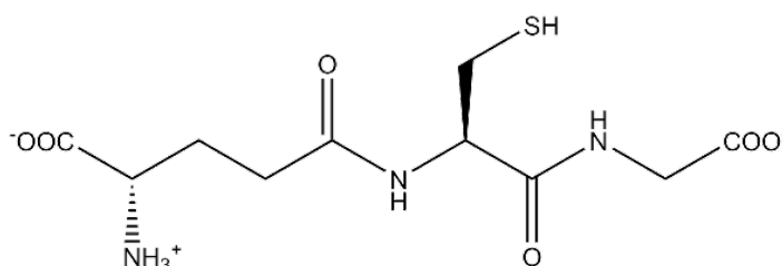
Глутатион
