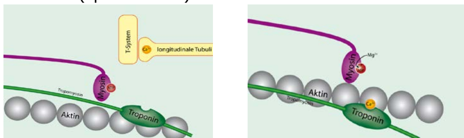
Рис. 2.6. Мышечное сокращение
