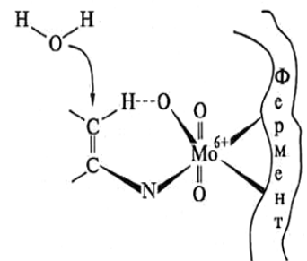
Нитратредуктаза, активный центр
