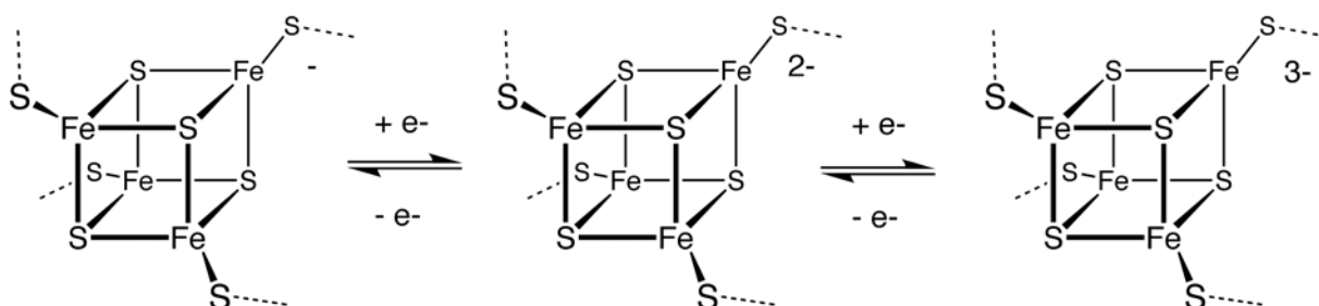
Пример железосерного кластера со структурой 4Fe-4S и его способность принимать электроны
