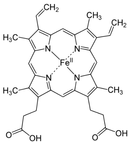
Гем (Fe(II) протопорфирин)
