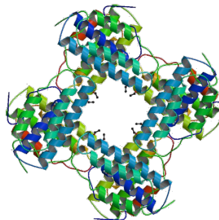
Гемэритрин
