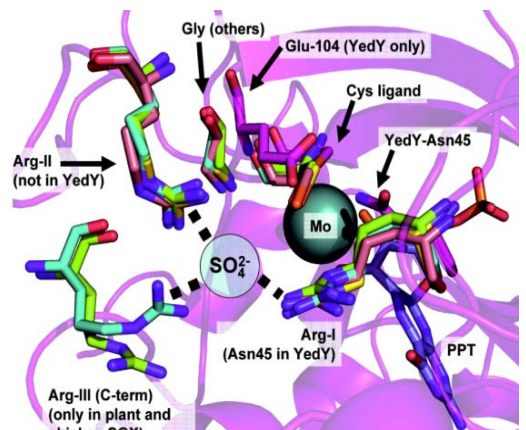
Сульфитоксидаза
