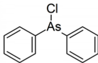
дифенилхлорарсин
