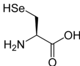
Селеноцистеин
