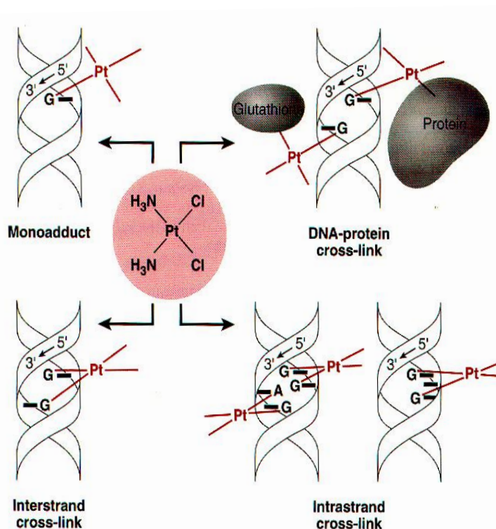
Рис. 12.2. «Платиновый аддукт»
