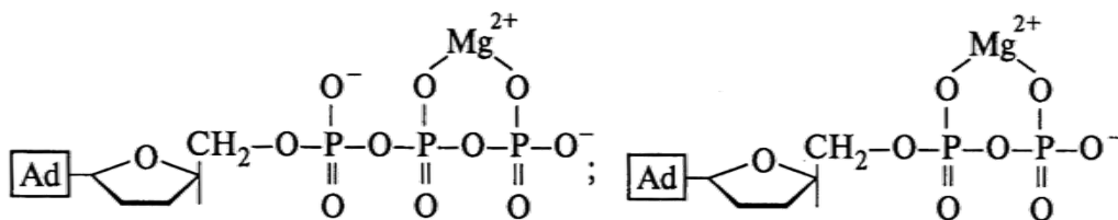
Рис. 2.4. Аденозинтрифосфат и аденозиндифосфат магния
