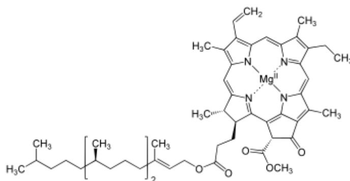
Хлорофилл а
