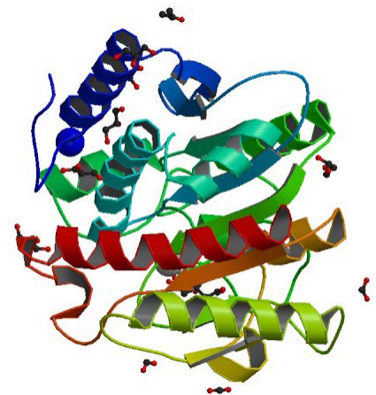
Карбоксипептидаза А
