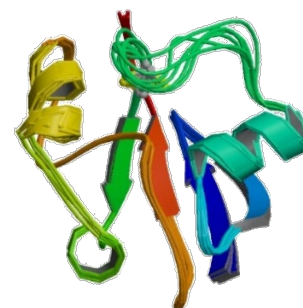
Путидаредоксин
