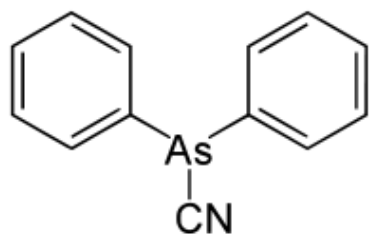
дифенилцианарсин
