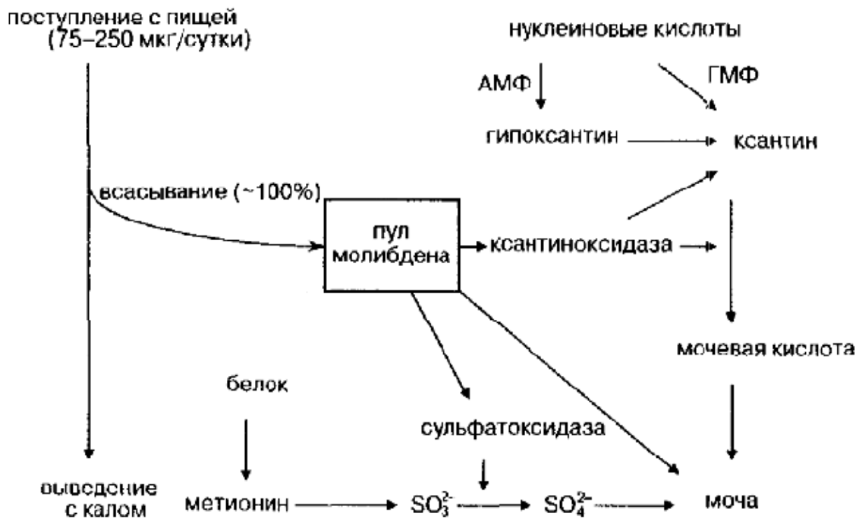
Рис. 12.3. Схема метаболизма молибдена в организме человека
