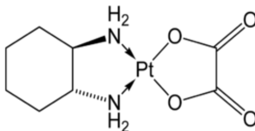
Оксалиплатин
