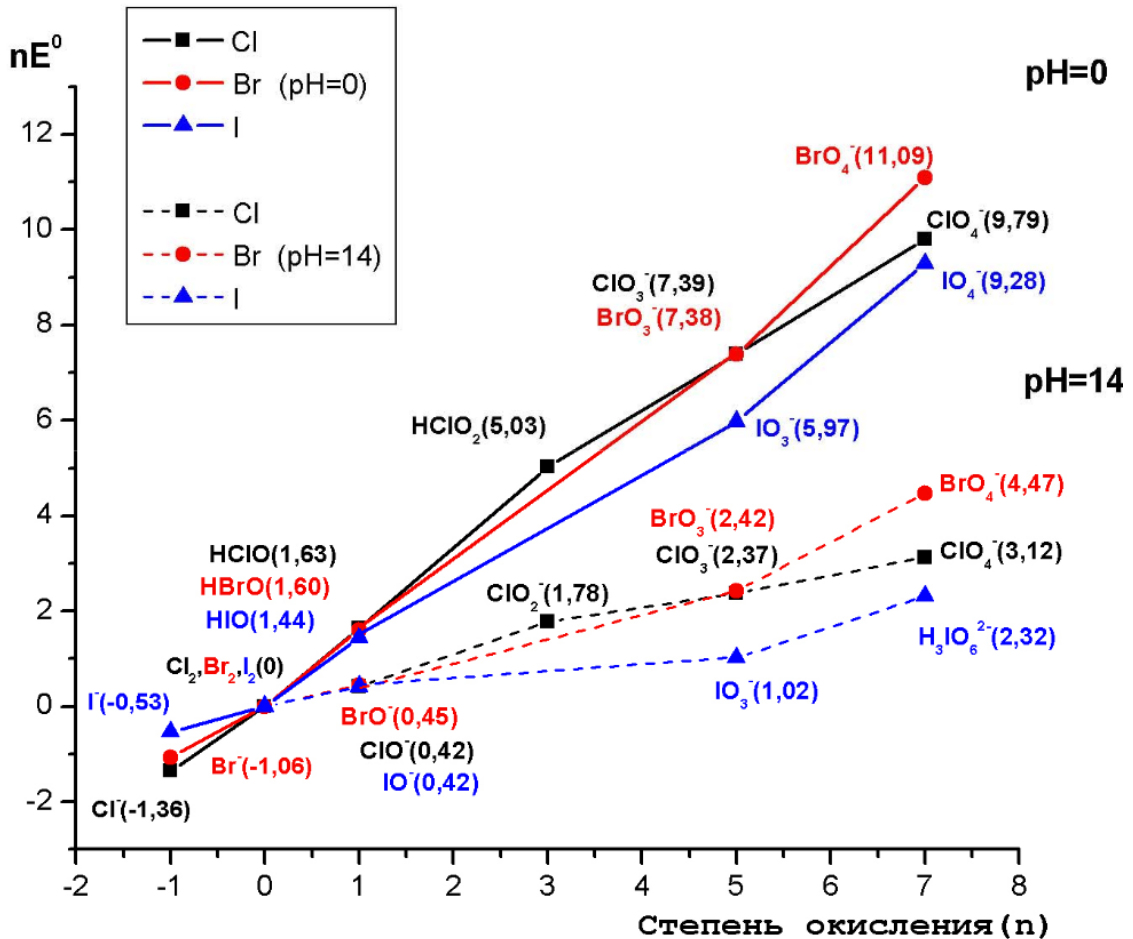
Рис. 7.1. Диаграмма Фроста для галогенов
