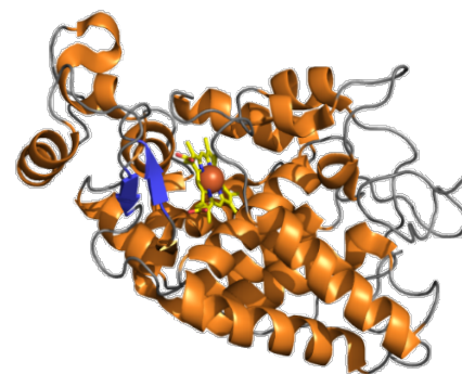
Пероксидаза хрена
