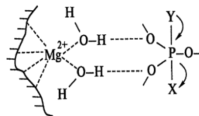
Фосфоглюкомутаза
