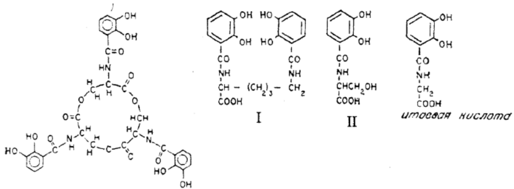
Энтеробактин
