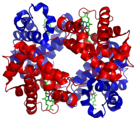
Гемоглобин
