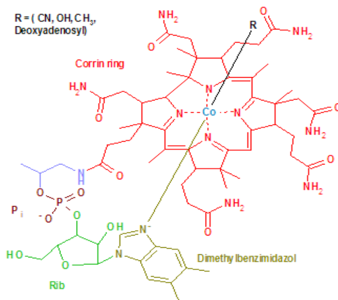
Витамин В 12
