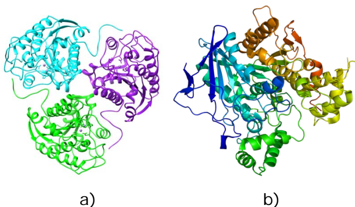
Рис. 11.6. Аргиназа (а); холинэстераза (b)
