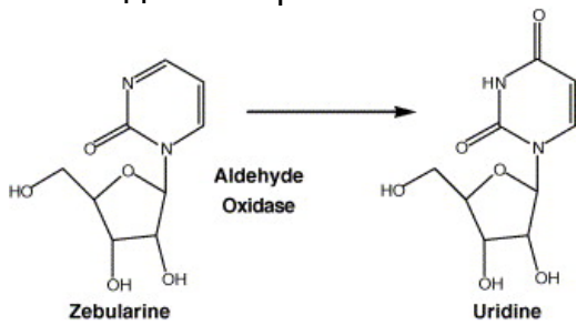
Рис. 12.5. Действие альдегидоксидазы на зебуларин
