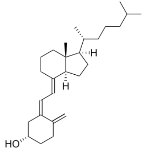
Холекальциферол (витамин D)
