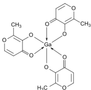
Малтолат галлия
