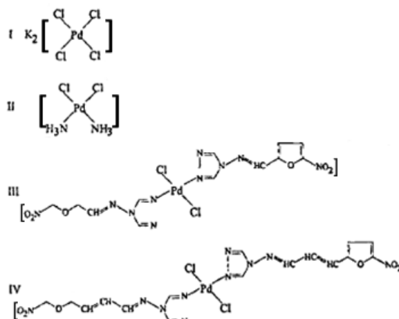
Рис. 12.1. Координационные соединения палладия
