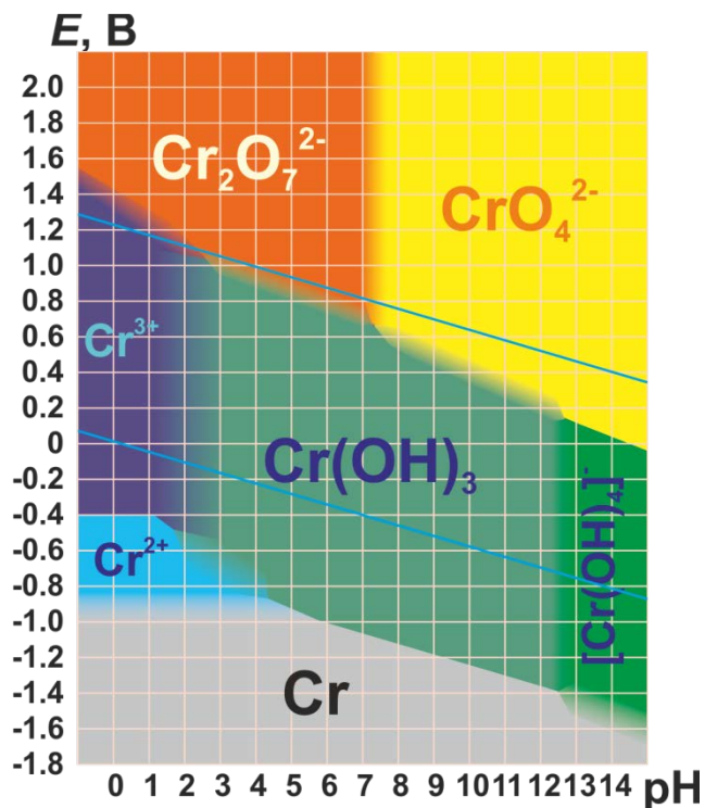
Рис. 11.3. Диаграмма pH-E для соединений хрома при 25°C
