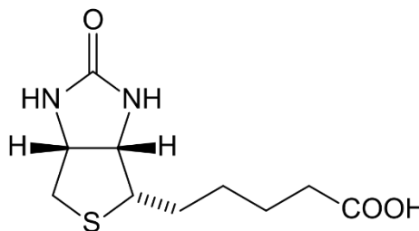
Биотин
