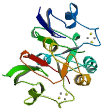
Адреноксин
