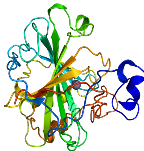
Карбоангидраза
