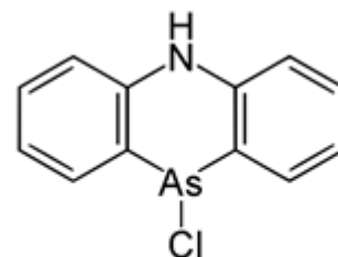
адамсит
