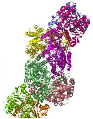
Нитрогеназа
