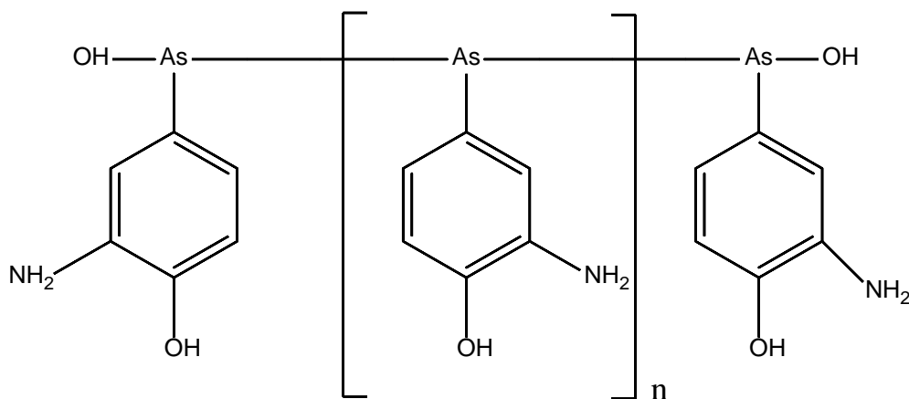
Рис. 5.4. Полимерное строение сальварсана
