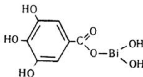
дерматол
