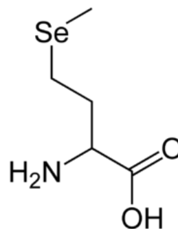
Селенометионин
