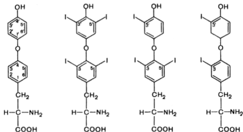
Рис. 7.6. Структура гормонов щитовидной железы (слева направо): тиронин; тироксин; трийодтиронин; дийодтиронин
