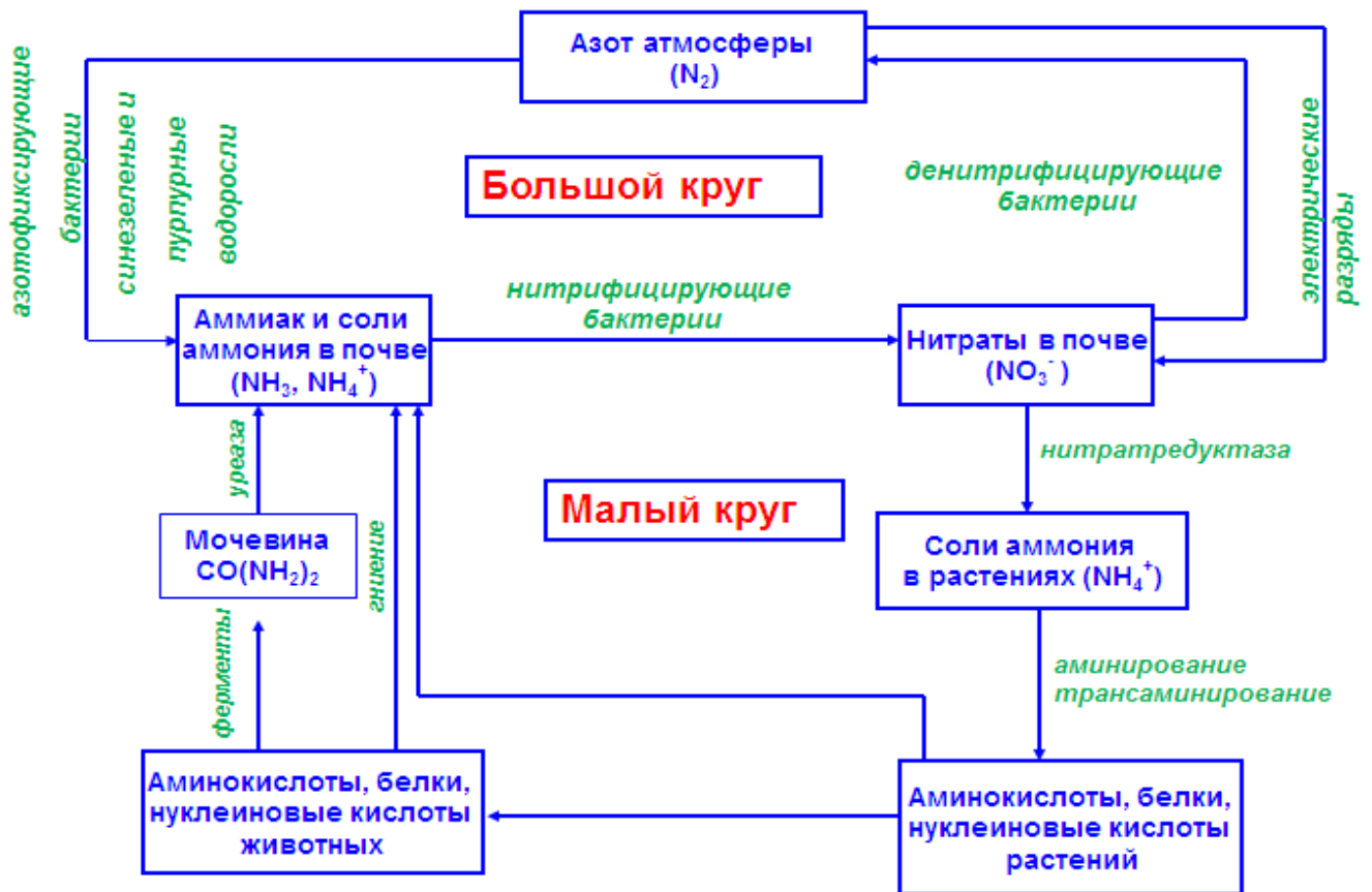
Рис. 5.2. Схема круговорота азота в природе
