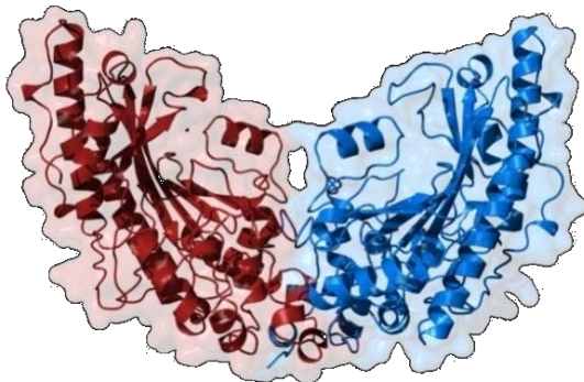
Тип M-S-E (креатинкиназа)
