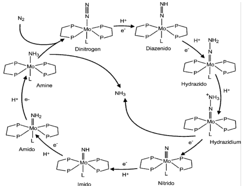
Рис. 12.4. Восстановление молекулярного азота нитрогеназой
