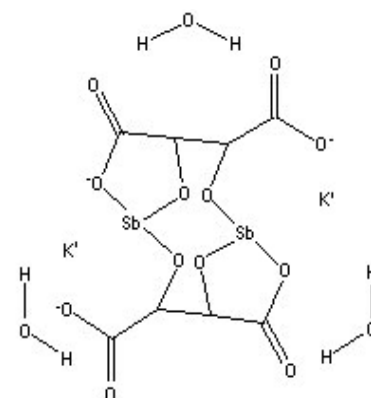
K_2Sb_2(OC_4H_4O_6)_2 \cdot 3H_2O Рвотный камень
