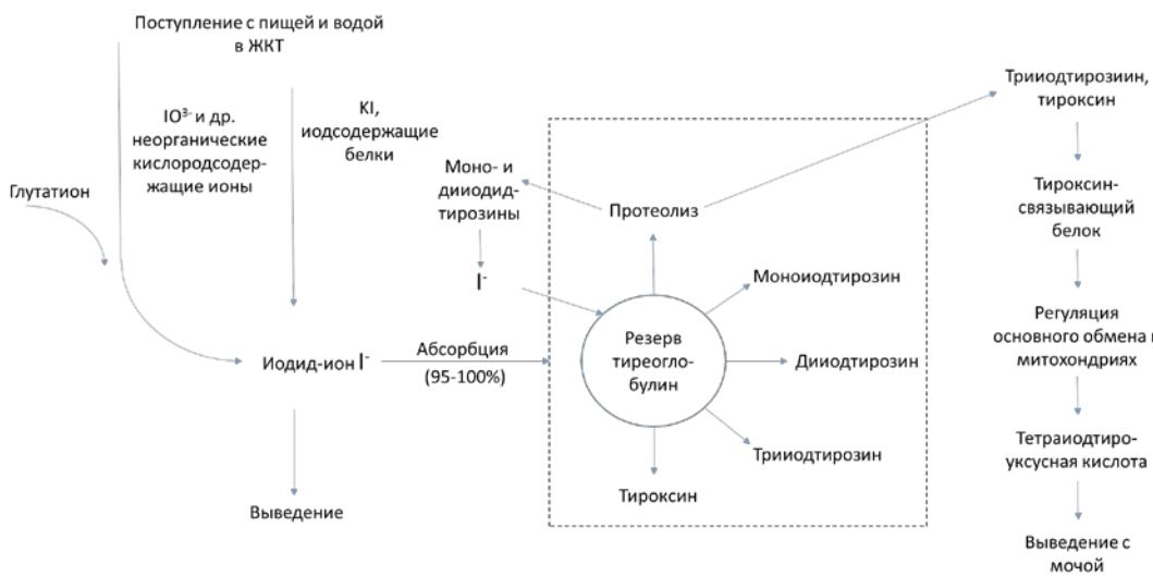
Рис. 7.5. Схема поступления и выведения иодид-ионов в организме
