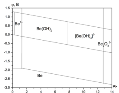
Рис. 2.1. Диаграмма "рН-потенциал" бериллия.
