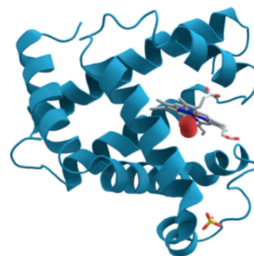
Миоглобин
