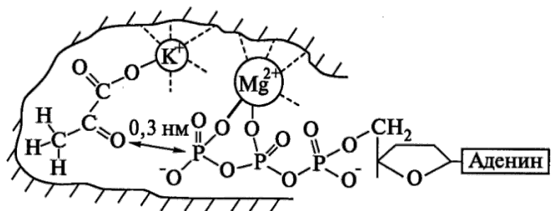
Тип S-M-E (пируваткиназа)
