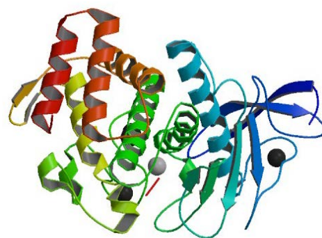
Термолизин
